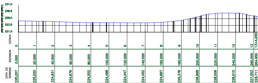
01 PERFIL LONGITUDINAL RUA FRANCISCO B. DE ALMEIDA - VARZEA DA BENTA S/ESC.
